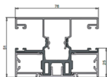
VISTA XT 76x51 doppelt
