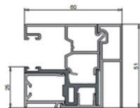
VISTA XT 60x51 einfach ALU
